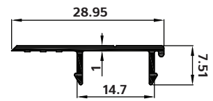
P-107936 ฝาตบเฟรมข้าง
