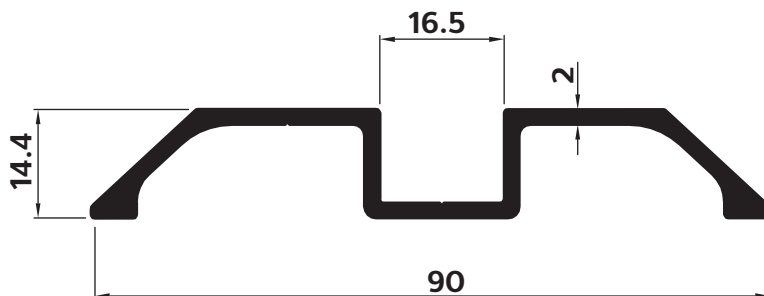
P-208901 เฟรมจกบ ล่าง (ภายใน)
