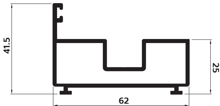
P-157935 เฟรมจกบ ล่าง (ภายนอก)
