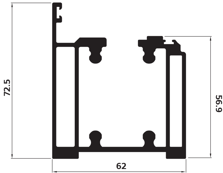
P-158907 เฟรมจกบ บน-ข้าง
