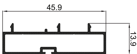
P-003588 ฝาครอบบาน ด้านล่าง
