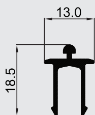
P-103104 ប្រព័ន្ធបង្ហូរ ER
