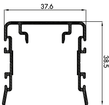
P-133106 ตบเกี่ยว 2 ทาง ร่องสีกหลาดคู่
