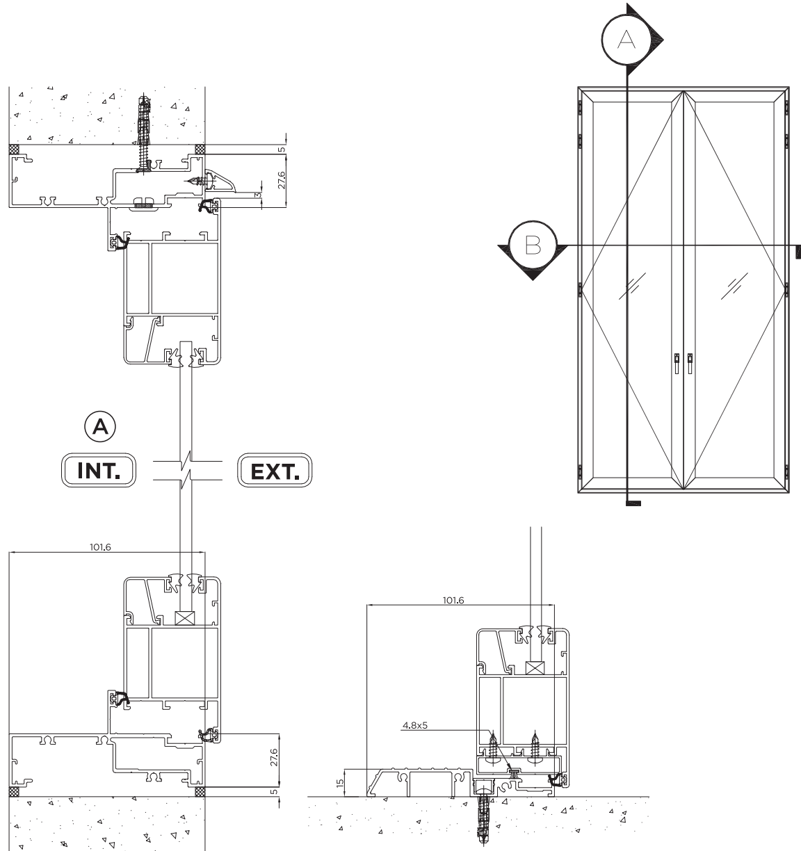
เฟรมบาน-ล่าง หน้าต่าง ขนาด 4"
