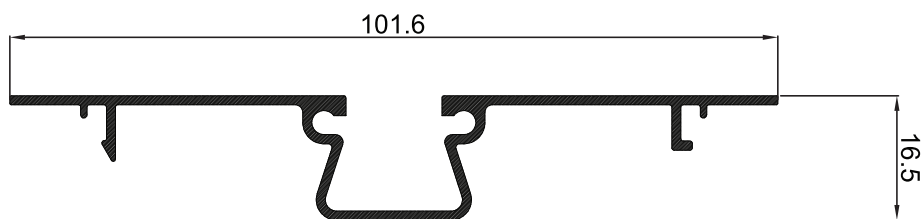
P-003093 ถပ်ร่องขยยว ER
