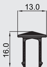
P-009511 ប្រព័ន្ធបង្ហូរ បង្ហូរ-ស្រោច
