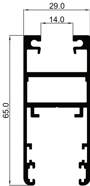
P-007229 กรอบบานมัลติล็อก ER
