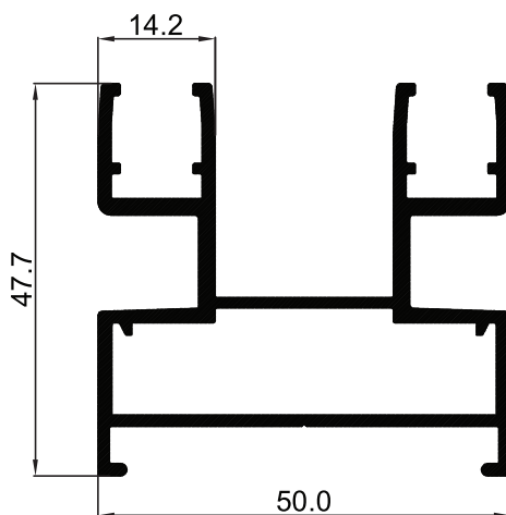
P-009519 ប្រព័ន្ធបង្ហូរ 2 ជាន់
