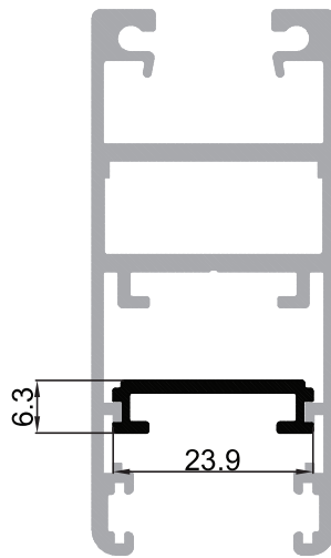
P-007227 ซีลรีบบาน ER
