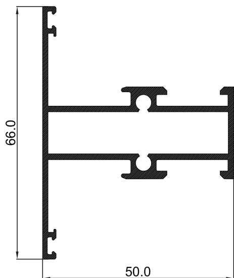
P-007225 แบ่งบาน ER
