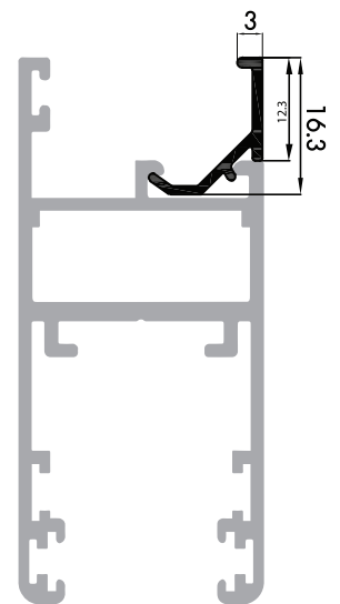
P-123119 คิ้ว (ระยะ 20 มม.)
