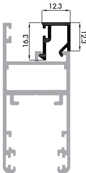
P-007227 ซีลรีบบาน ER
