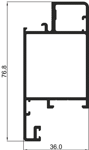
P-003598 กรอบบาน
