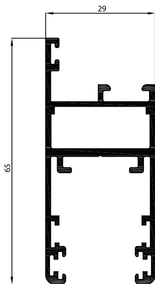
P-007229 กรอบบานมัลติล็อก ER
