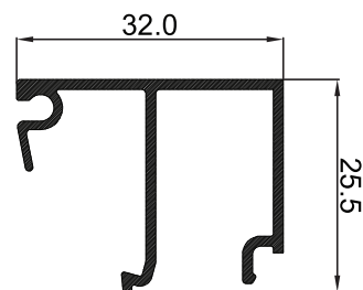
P-006061 คิ้วเหลี่ยม ER
