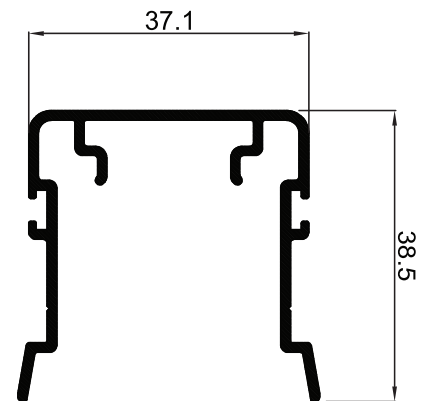
P-003695 ตบเกี่ยวสองด้าน
