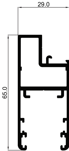
P-003590 กรอบบาน
