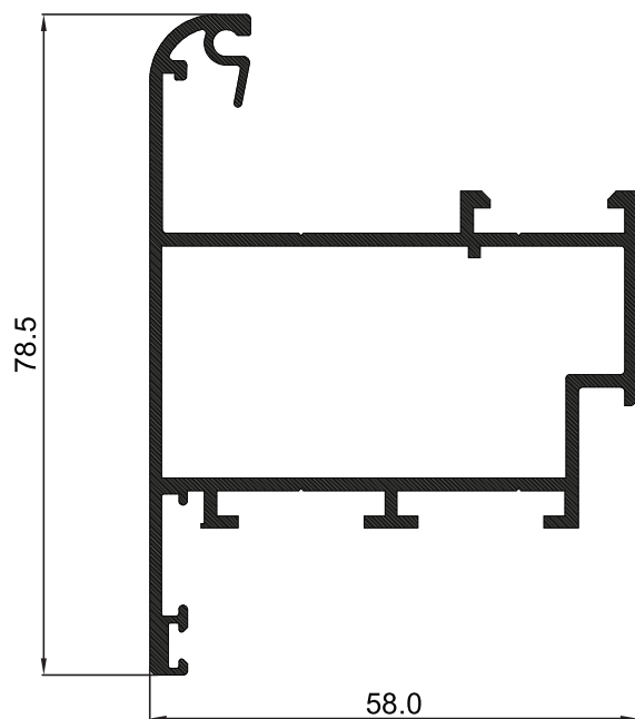
P-009517 กรอบบานหน้าต่าง ER
