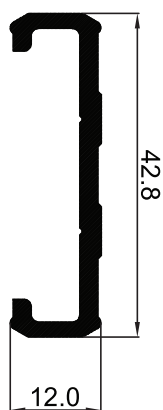
P-009413 ไส้ต่อบาน fix
