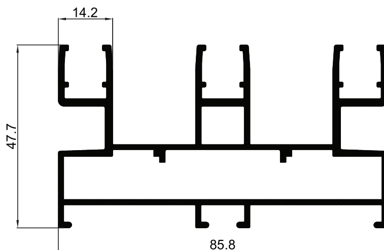
P-009509 ប្រព័ន្ធបង្ហូរ 3 ជាន់
