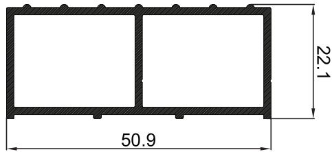
P-003599 เฟรมล่าง
