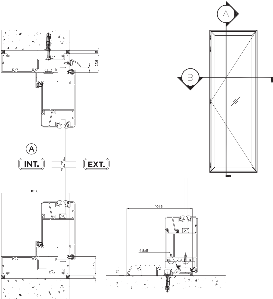
เฟรมบาน-ล่าง หน้าต่าง ขนาด 4"
